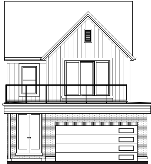
ELEVATION A
